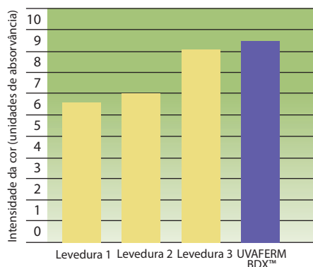
Intensidade corante os vinhos fermentados em Syrah Claire Valley, Instituto Australiano de Investigação do Vinho
