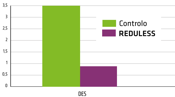
Figura 1: Concentração ( \mu\text{g/L} ) de Dietilsulfato (DES) em vinho tinto antes e após a aplicação do REDULESS .
